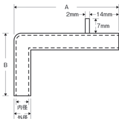
【L型寸法図】
