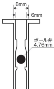
【8Φボール弁付断面図】
