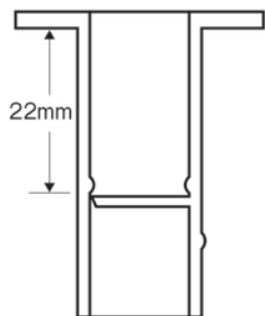
【逆流防止弁付断面図】
