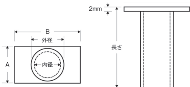
【T型寸法図】
