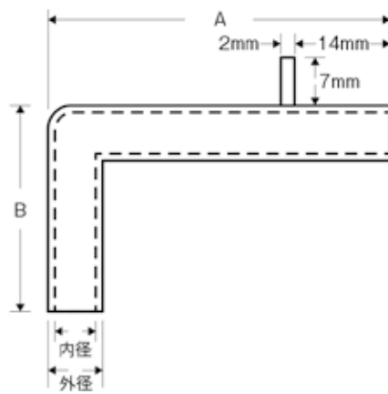
【L 型寸法図】
