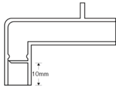
【逆流防止弁付きの断面図】
